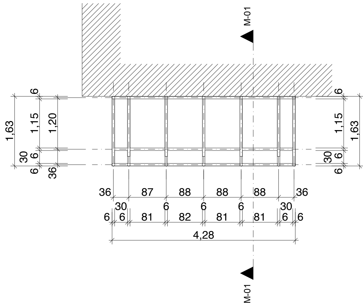
1. Tető terv 1:50
