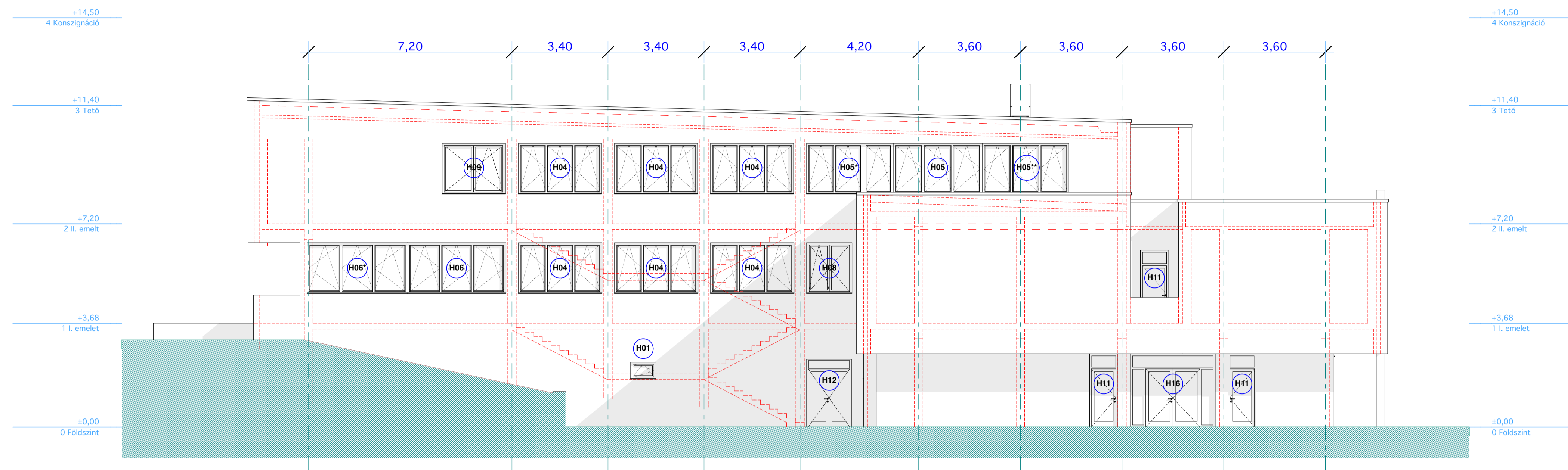
EK-i homlokzat 1:100
