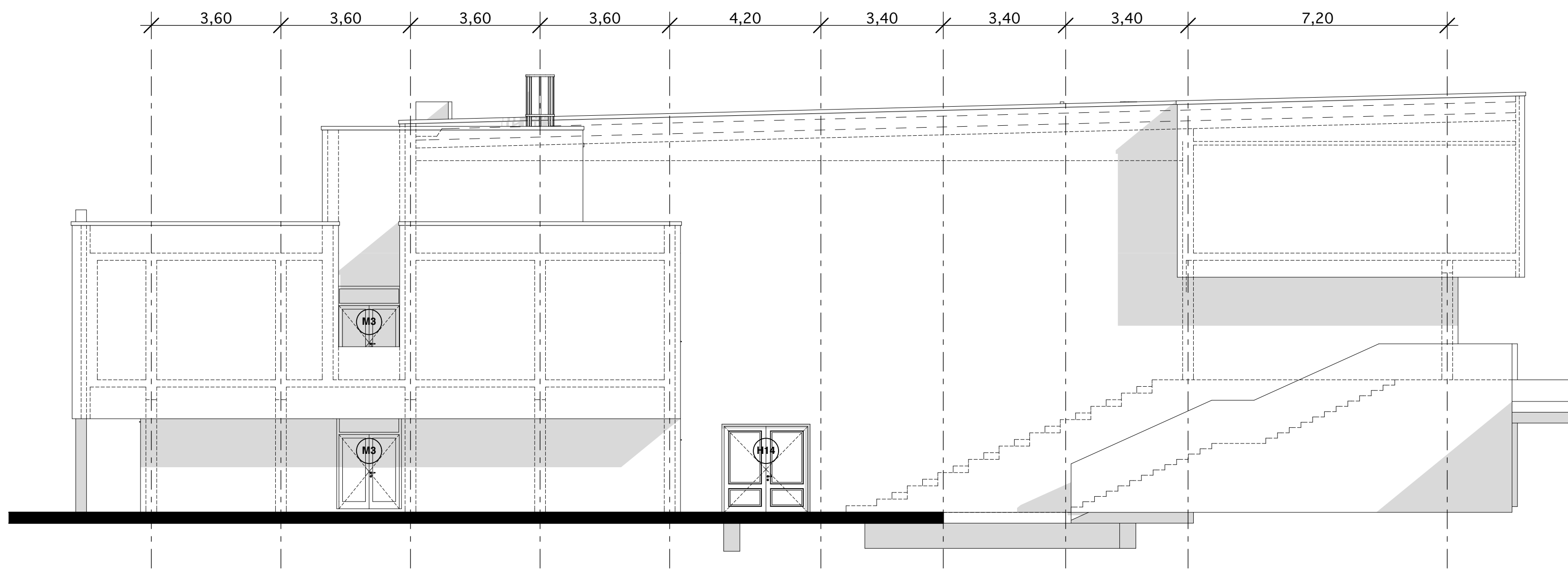
DNy-i homlokzat 1:100
